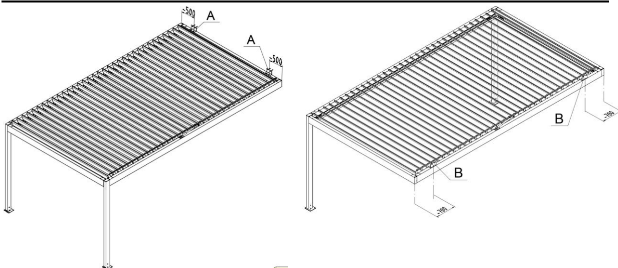
A – Uchwyty ściennie montowane do belek poprzecznych.
