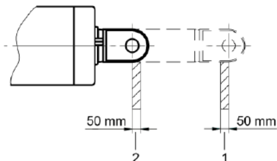
Rysunek 54 Dopuszczalna redukcja skoku silnika Picoło
